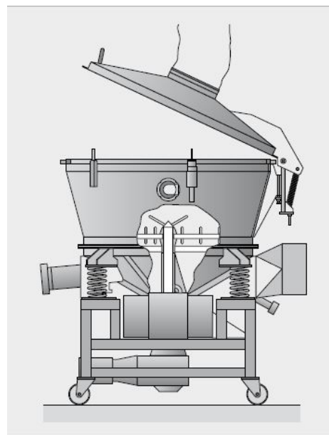
Рис. 99. Вибросушилка периодического действия: а ) общий вид, б ) схема сушилки
