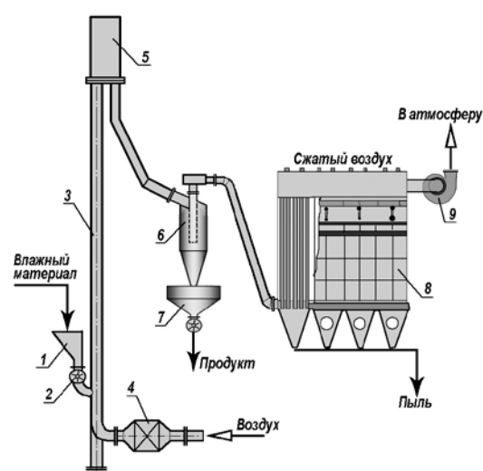
Рис. 78. Пневматическая сушилка: 1 - бункер, 2 - питатель, 3 - труба; 4 - калорифер, 5 - сборник-амортизатор, 6 - циклон, 7 - бункер, 8 - фильтр, 9 - вентилятор
