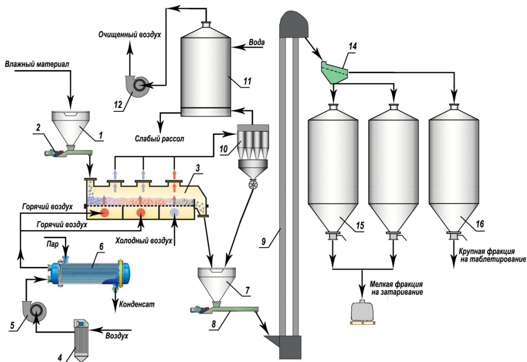
Рис. 69. Схема сушки поваренной соли в сушилке взвешенного слоя:
