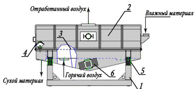
Рис. 70. Вибрационная конвективная сушилка. 1 - рама; 2 - крышка; 3 - перфорированный лист (решетка); 4 - заслонка; 5 - пружины; 6 - вибропривод.
