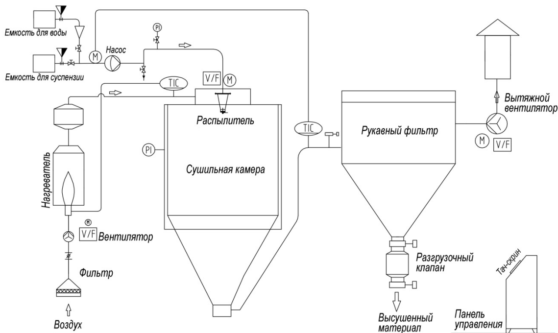
Рис.77. Технологическая схема сушки.
