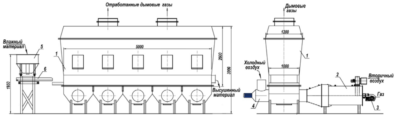
Рис. 104. Схема сушилки КС:
