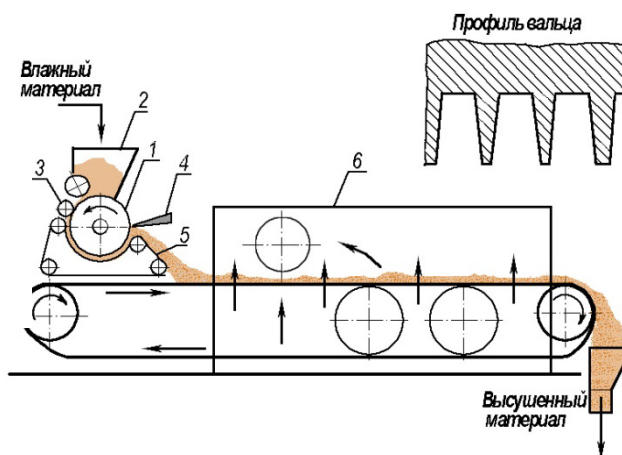
Рис. 90. Одновальцовая формующая сушилка:
