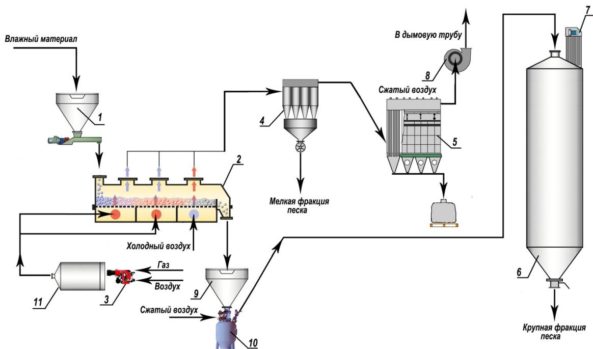
Рис. 103. Технологическая схема сушки карьерного песка в сушилке КС:
