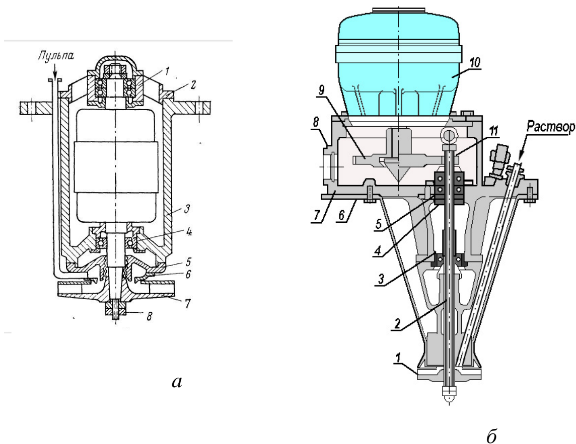
Рис.76. Конструкция распылителей:
