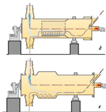
Рис. 62. Барабанные сушилки: д – с мелющими телами, е – с камерой для обеспыливания материала
