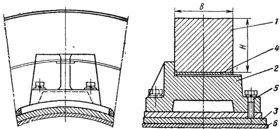
Рис. 57. Башмак для крепления бандажа: 1 - бандаж, 2 - башмак, 3 - усиление обечайки, 4 - прокладка, 5 - болты, 6 - обечайка барабана
