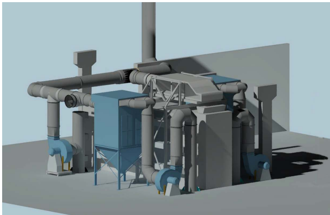
Рис. 114. Ленточная сушилка – общий вид
