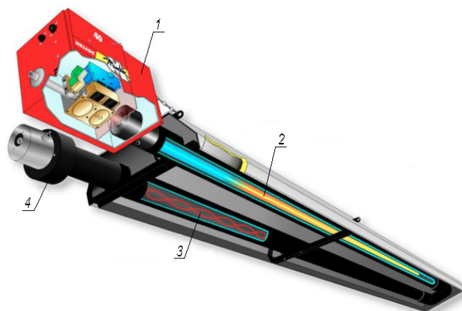
Рис. 93. Газовый ИК-излучатель: 1 – газовая горелка, 2 – теплоизлучатель; 3 – завихритель, 4 – вентилятор
