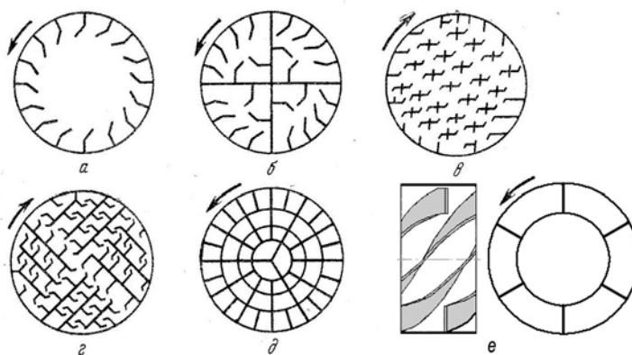
Рис. 55. Типы насадок барабанных сушилок:
