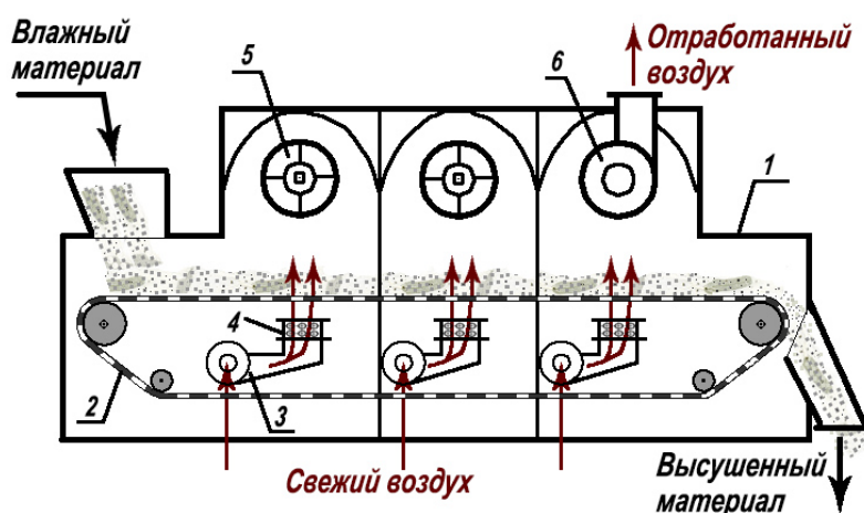
Рис. 50. Ленточная сушилка:
