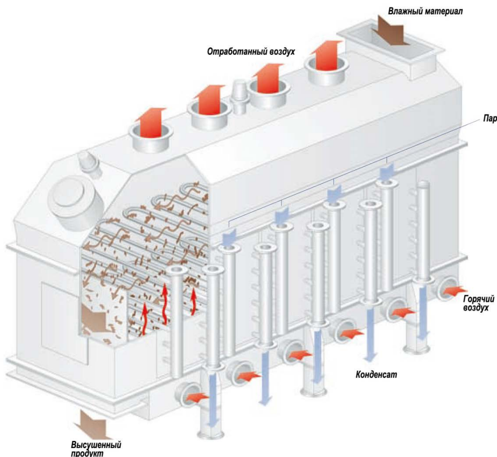
Рис. 108. Схема сушилки взвешенного слоя с подогревом воздуха внутри сушильной камеры
