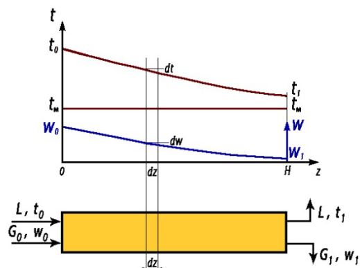
Рис. 43. Изменение температуры сушильного агента t , влажности материала w для непрерывной прямооточной сушилки
