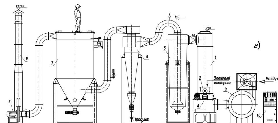
Рис. 79. Флеш-сушилка:
