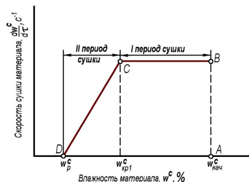
Рис. 44. Упрощенное представление кривой сушки
