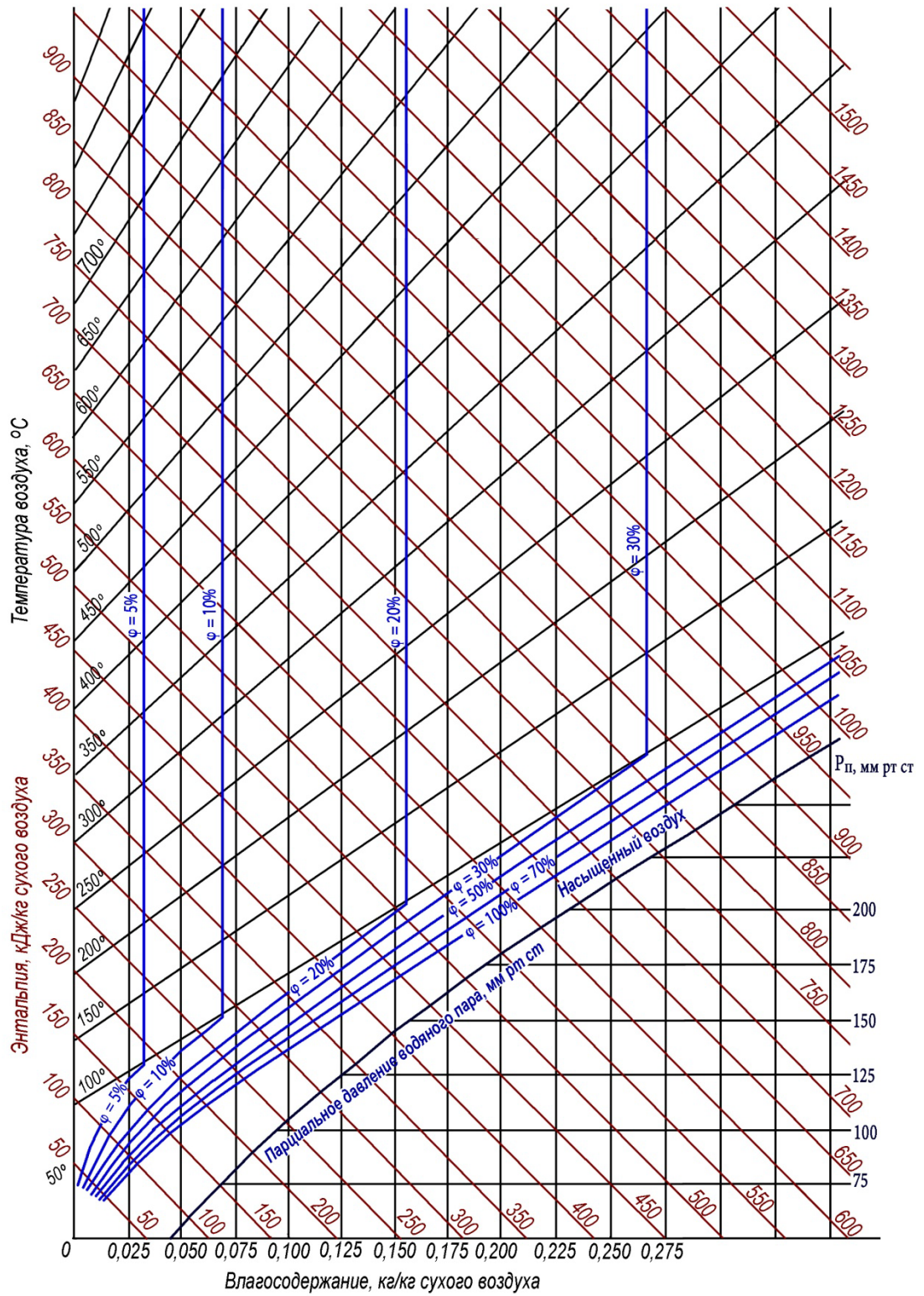
Рис. 7. Диаграмма I - x для влажного воздуха
