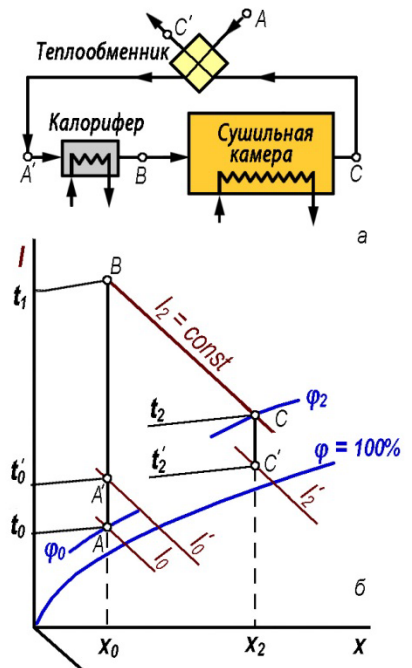
Рис. 21. Сушилка с рекуперацией тепла отходящих газов: а – принципиальная схема, б – изображение теоретического процесса на диаграмме.
