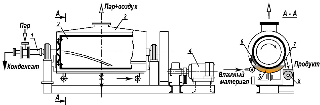
Рис. 87. Одновальцовая сушилка: 1-полая цапфа; 2- валец; 3-вытяжной зонт; 4- привод; 5- корыто; 6- калибрующее устройство; 7- скребковое устройство; 8- шнек
