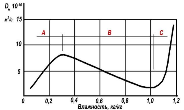
Рис. 41. Изменение коэффициента влагопроводности D_M ( \text{м}^2/\text{с} ) древесины (сосна) от ее влажности при температуре 30^\circ\text{C}
