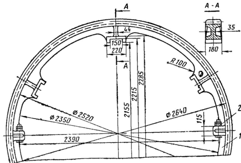
Рис. 59. Венцовая шестерня:
