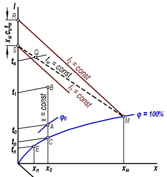
Рис. 9. Изображение изменения состояния влажного воздуха на I - x диаграмме.
