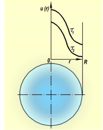
Рис. 33. Зависимость влажности от координаты r и \tau при сушке шара
