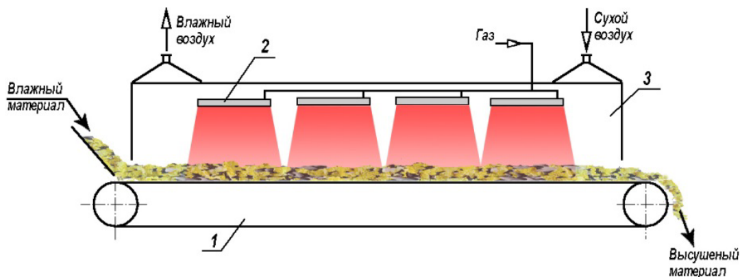
Рис. 94. Терморрадиационная сушилка с газовыми ИК-излучателями: 1 – транспортерная лента, 2 – газовые излучатели; 3 – кожух сушильной камеры
