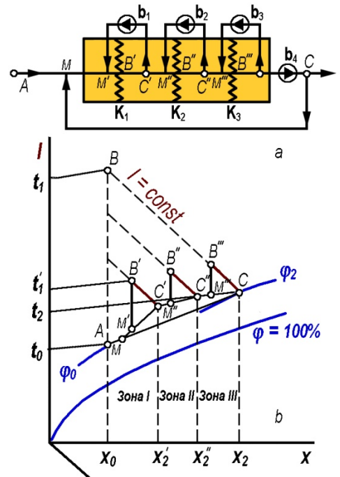
Рис. 20. Сушилка с промежуточным подогревом и рециркуляцией воздуха по зонам: а – принципиальная схема, б – изображение теоретического процесса на диаграмме.
