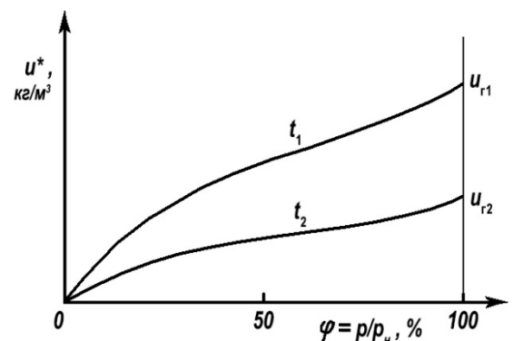
Рис. 32. Изотермы равновесия влажного материала
