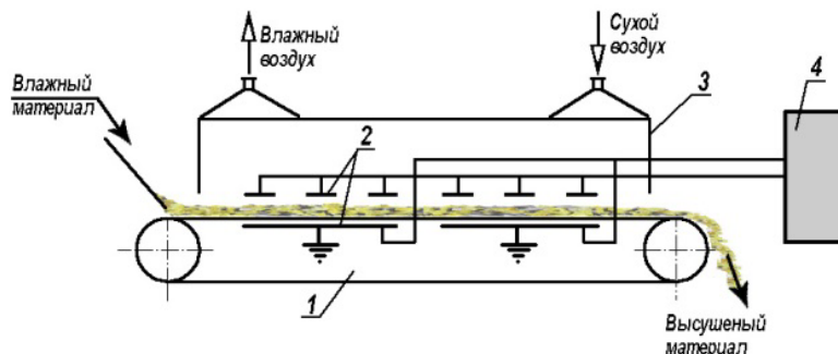
Рис. 95. Высокочастотная (диэлектрическая) сушилка:
