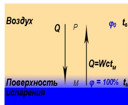
Рис.10. Схема адиабатического испарения влаги с поверхности воды
