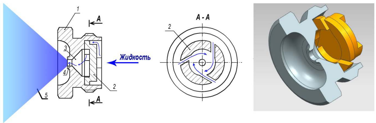
Рис.74. Центробежная форсунка:
