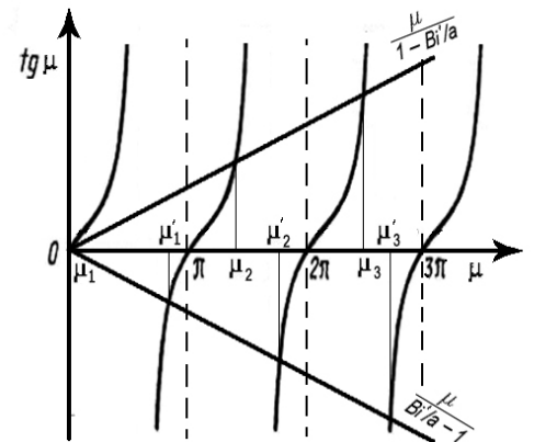
Рис. 34. Корни \mu характеристического уравнения (6.50)
