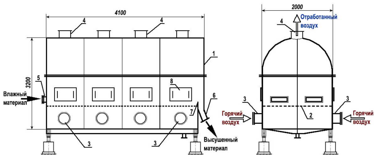
Рис. 65. Четырех секционная сушилка с кипящим слоем материала:
