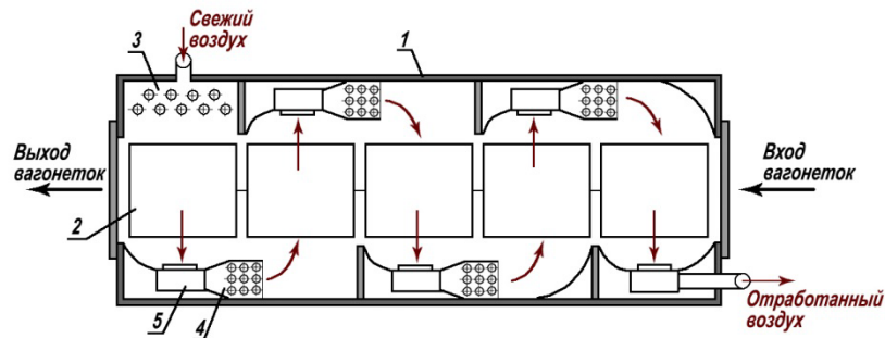
Рис. 49. Туннельная сушилка: 1 – сушильная камера, 2 - вагонетки, 3 – основной калорифер, 4 – дополнительные калориферы, 5 - вентиляторы
