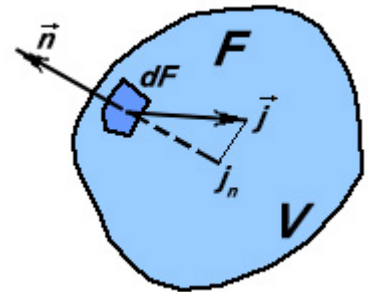
Рис. 29. К выводу уравнения переноса влаги внутри влажного материала
