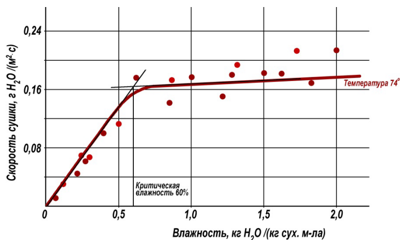
Рис. 116. Экспериментальная кривая скорости сушки для стружки осины (а), фото стружки (б)
