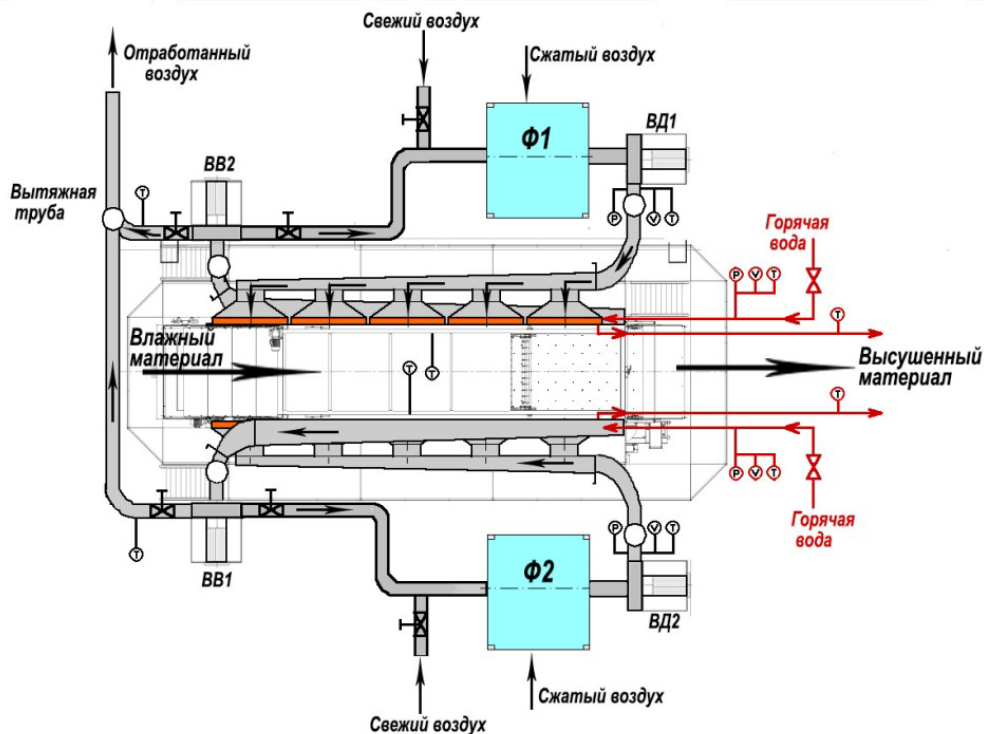
Рис. 53. Схема установки контрольных приборов на шестиярусной ленточной сушилке: ВД – дутьевые вентиляторы, ВВ – вытяжные вентиляторы, Ф – рукавные фильтры.
