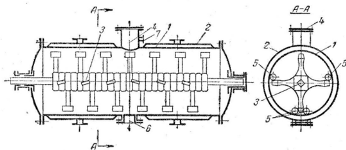
Рис. 82. Гребковая вакуум-сушилка: 1 - корпус сушилки, 2 - паровая рубашка, 3 - мешалка, 4 - загрузочный люк, 5 - трубы, способствующие перемешиванию материала, 6 - разгрузочный люк, 7- штуцер для присоединения к вакууму
