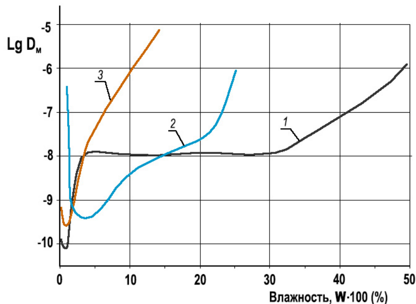
Рис. 42. Зависимость коэффициента влагопроводности D_M ( \text{м}^2/\text{с} ) от влажности 1 – газобетон, 2 – керамический кирпич, 3 – гипс
