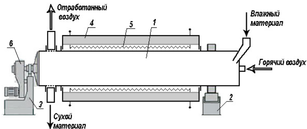
Рис. 92. Барабанная контактная сушилка:
