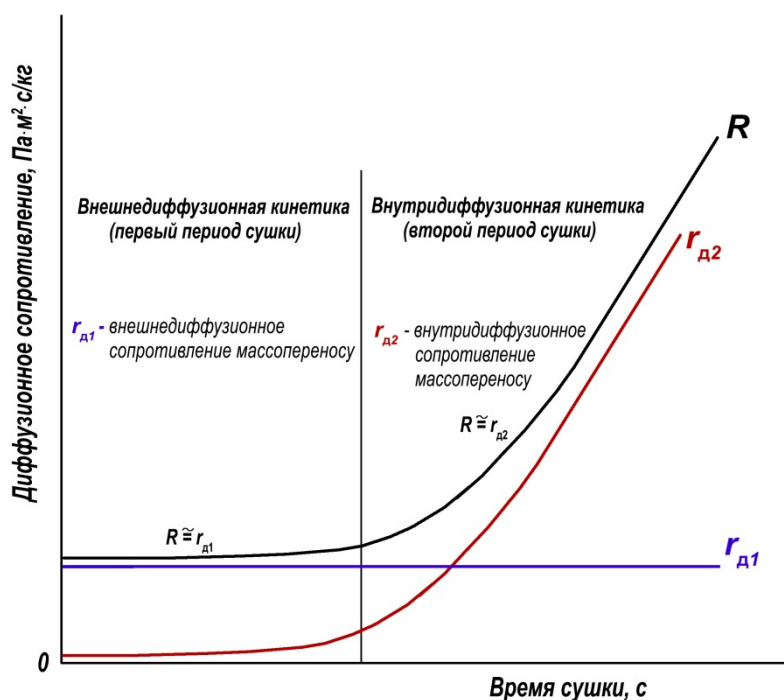
Рис. 24. Изменение диффузионных сопротивлений в процессе сушки влажного материала
