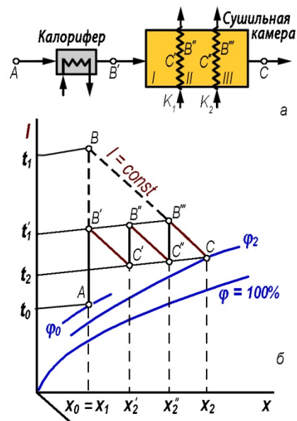
Рис 17. Сушилка с промежуточным подогревом воздуха по зонам: а – принципиальная схема, б - изображение на диаграмме
