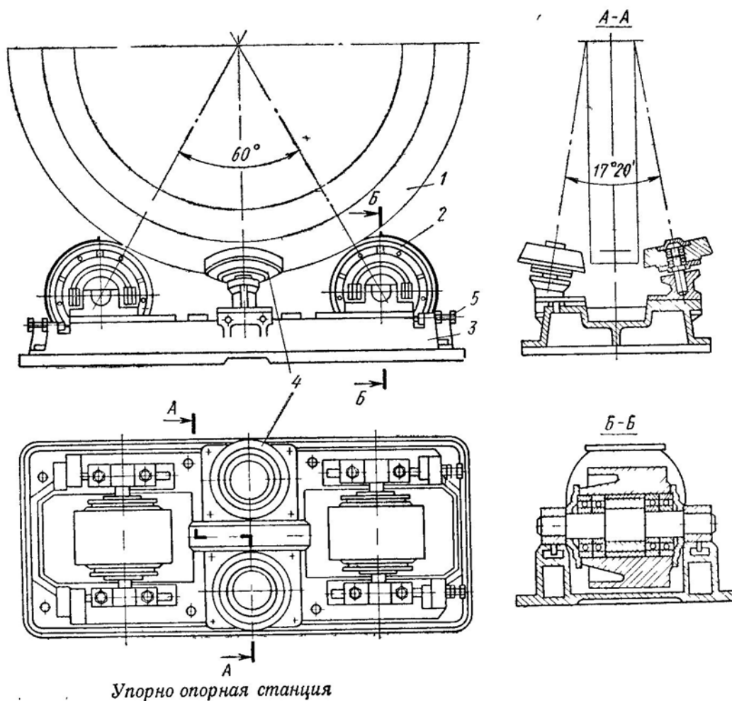
Рис. 58. Упорно-опорная станция: 1 - бандаж, 2 - опорные ролики, 3 - опорная рама, 4 - упорные ролики, 5 - регулировочные винты
