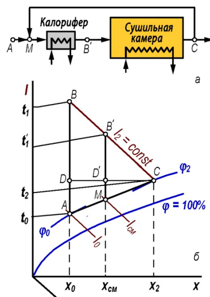
Рис. 19. Сушилка с частичной рециркуляцией отработанного воздуха: а – принципиальная схема, б – изображение теоретического процесса на диаграмме
