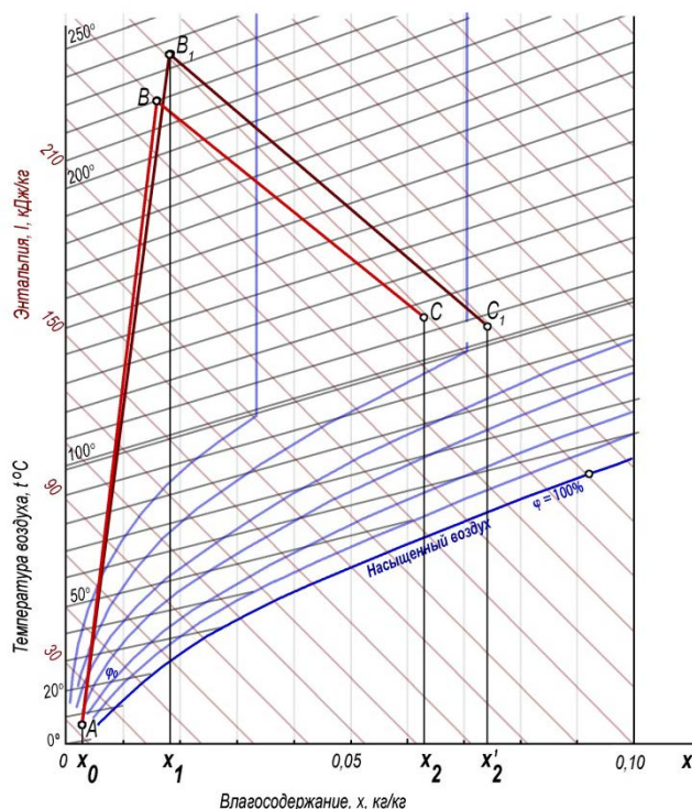
Рис. 110. Изображение процесса сушки пластификатора бетонов: ABC – исходный вариант, AB 1 C 1 –увеличение производительности
