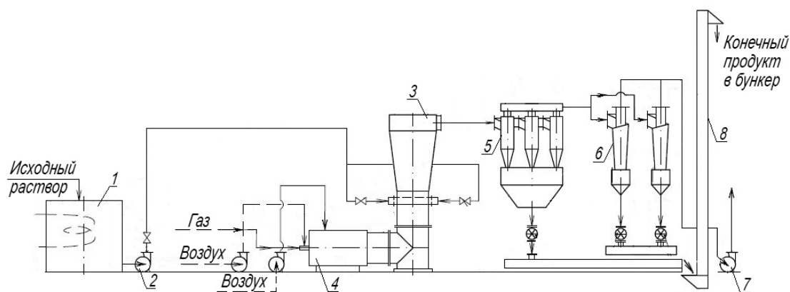
Рис. 109. Технологическая схема сушильной установки:
