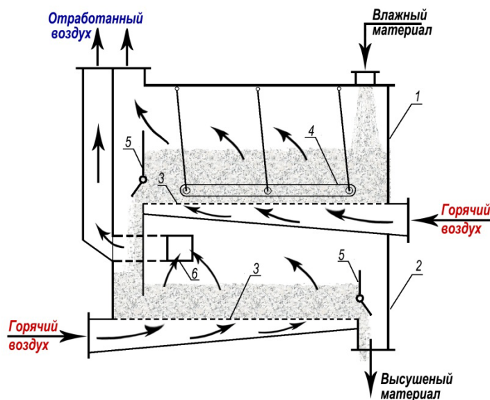
Рис. 66. Двухкамерная сушилка КС:
