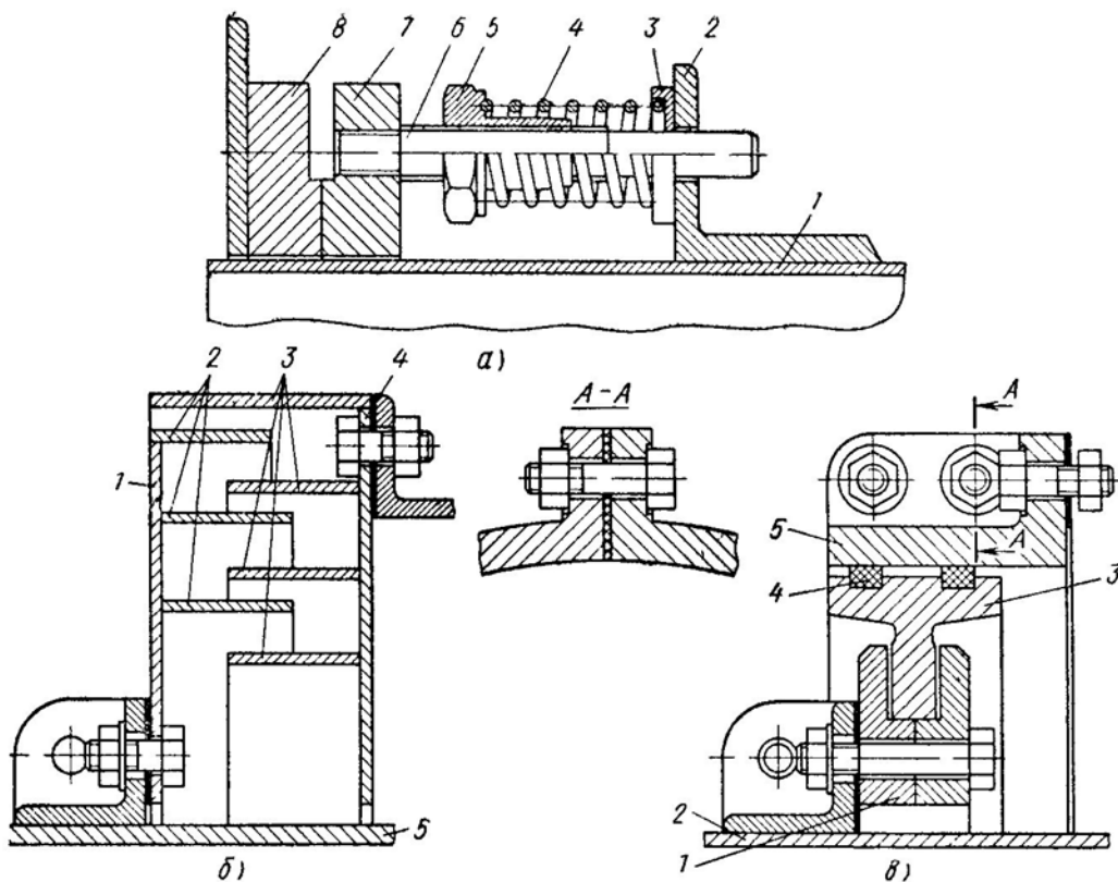
Рис. 60. Уплотнения барабана:
