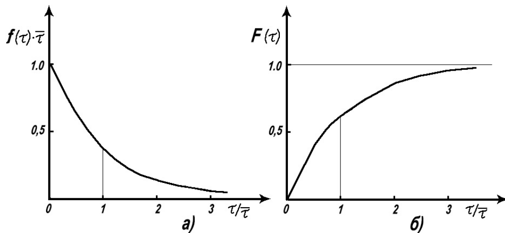
Рис. 45. Дифференциальная (а) и интегральная (б) функции распределения по времени пребывания частиц во взвешенном слое сушилки при режиме полного смешения
