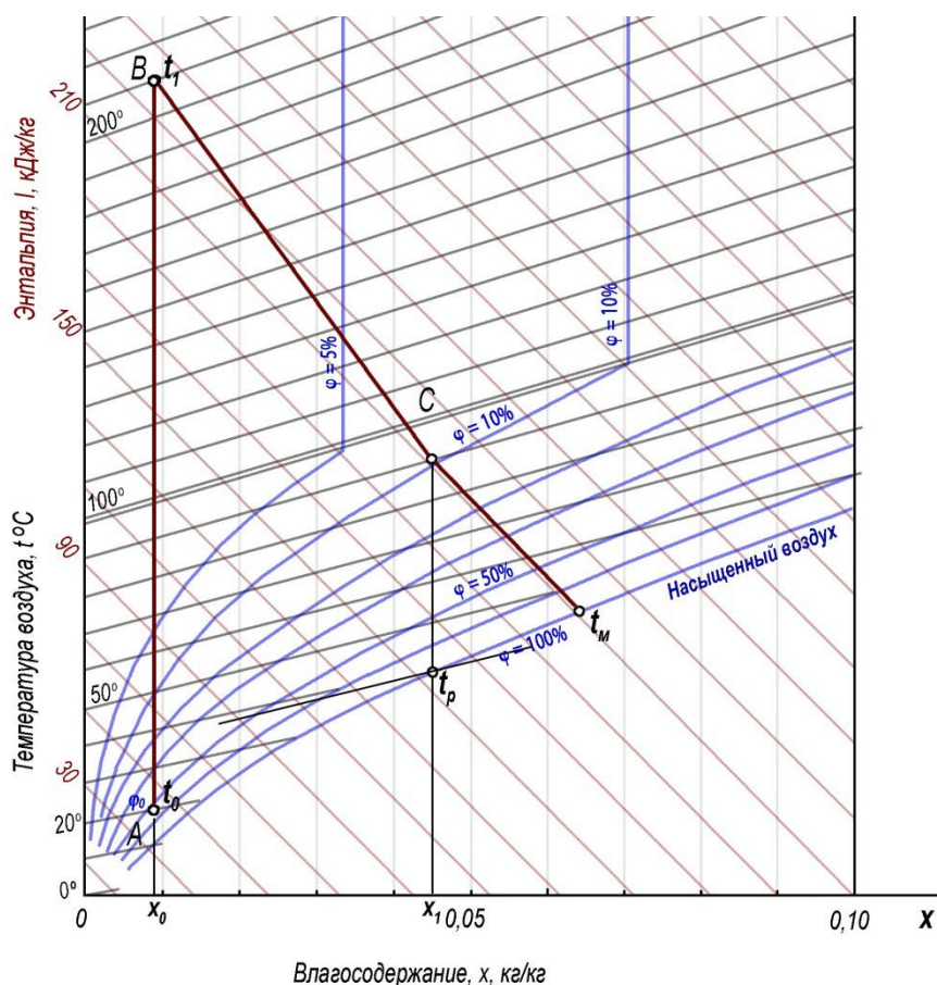
Рис. 112. Изображение сушки раствора ПВП в башенной распылительной сушилке: АВ – линия нагрева воздуха, ВС - линия сушки
