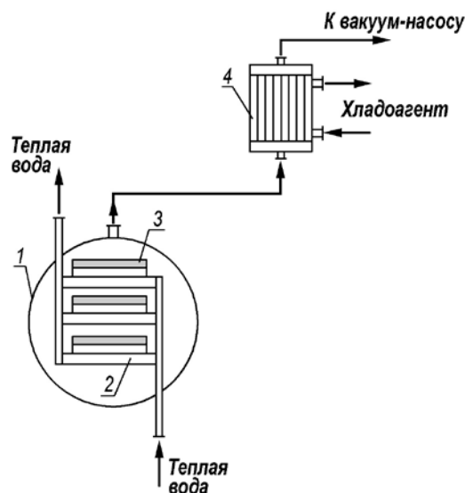
Рис. 97. Принципиальная схема сублимационной сушилки:
