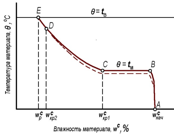
Рис. 28. Температурная кривая материала
