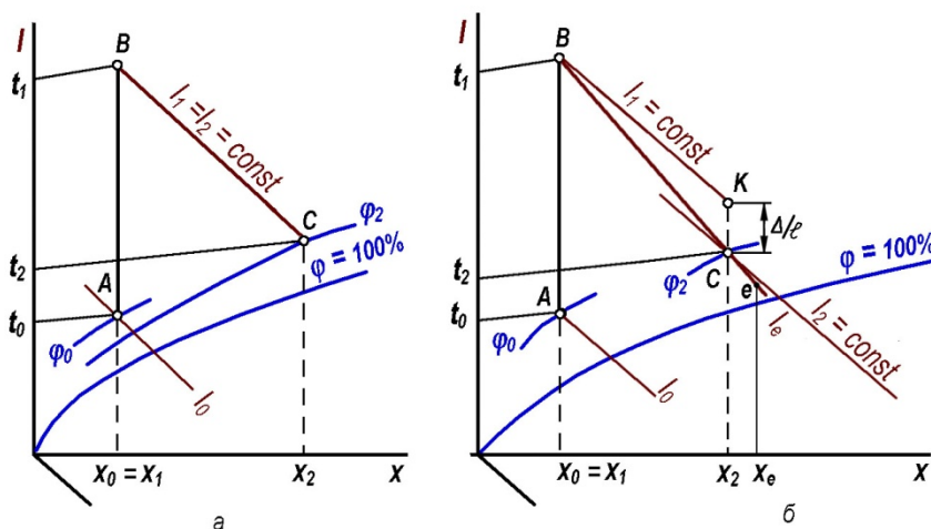
Рис. 15. Изображение процессов сушки на I - x диаграмме а - теоретическая сушилка, б - действительная сушилка
