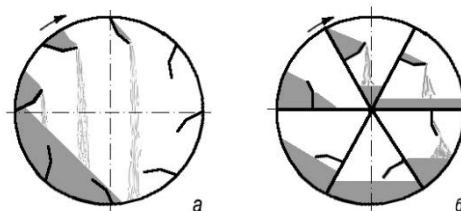
Рис. 56. Схема пересыпания материала: a – на подъемно-лопастной и б – на секторной насадке
