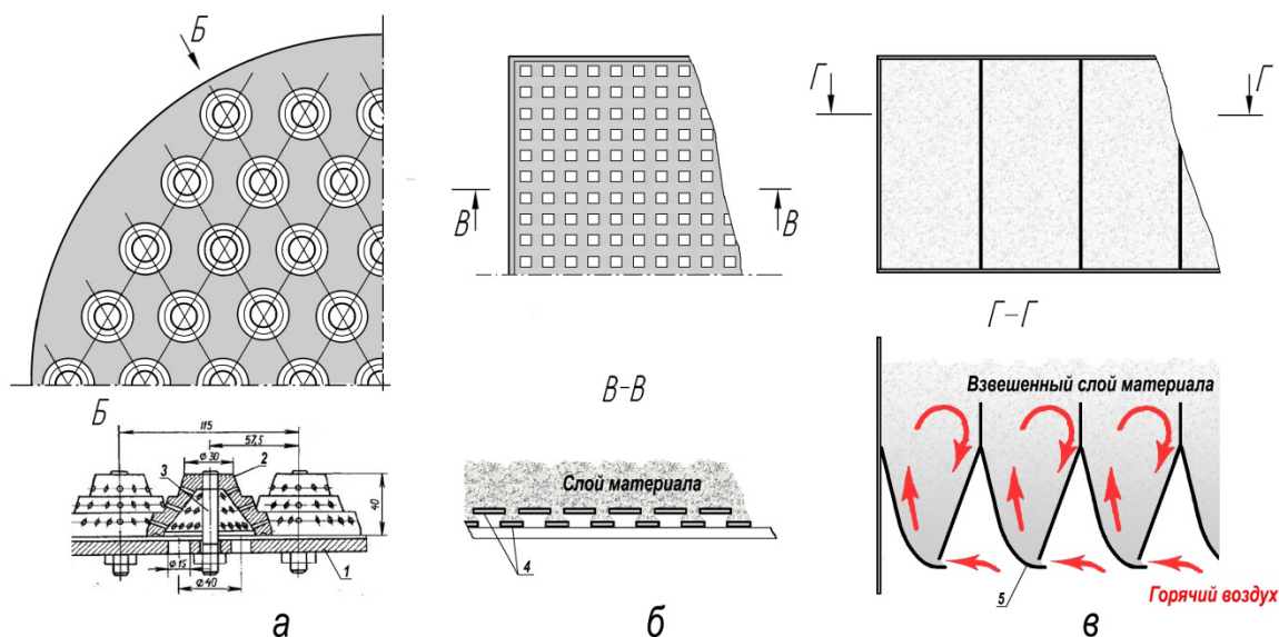
Рис. 68. Конструкция беспровальных газораспределительных решеток: а - колпачковая, б - двухслойная; в – вихревая.
