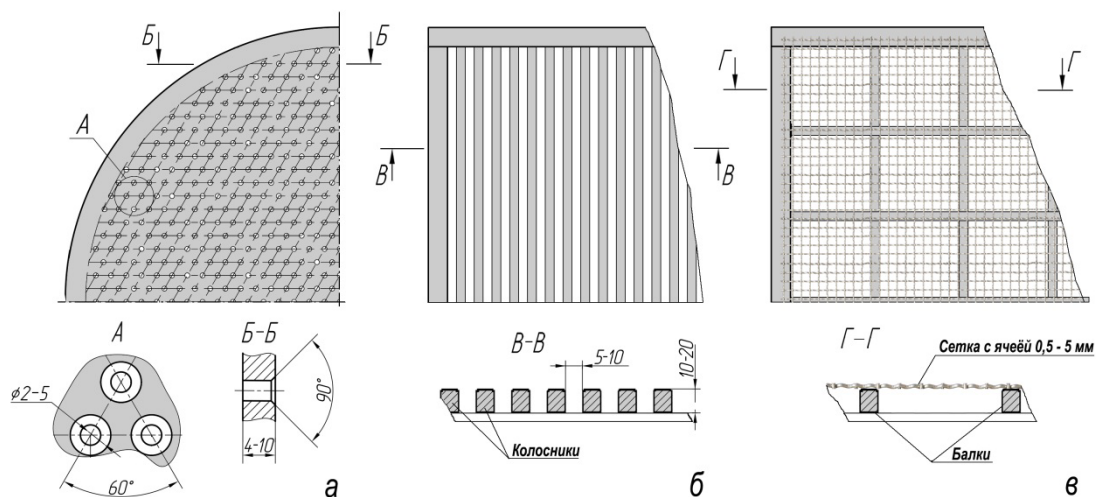
Рис. 67. Конструкция газораспределительных решеток: а - дырчатая, б - решетчатая; в – сетчатая
