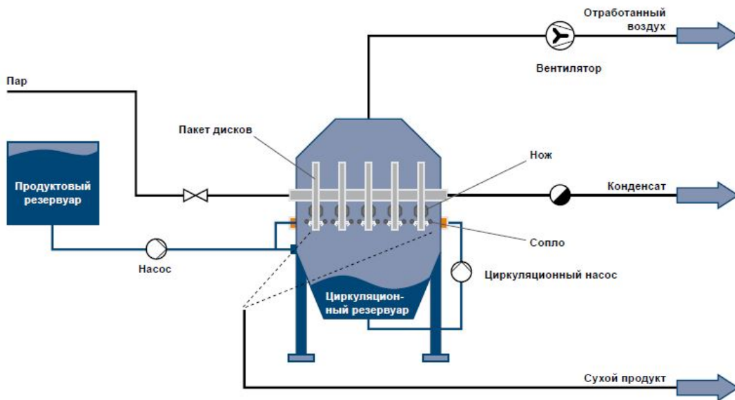
Рис. 91. Дисковая сушилка
