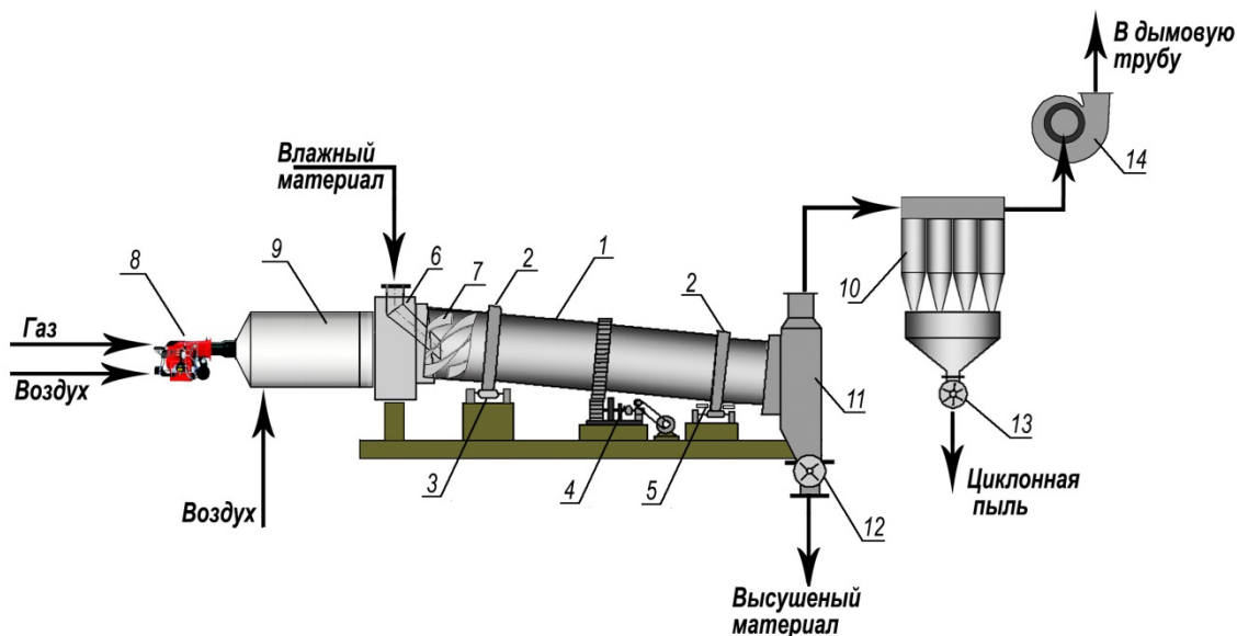
Рис. 54. Барабанная сушилка:
