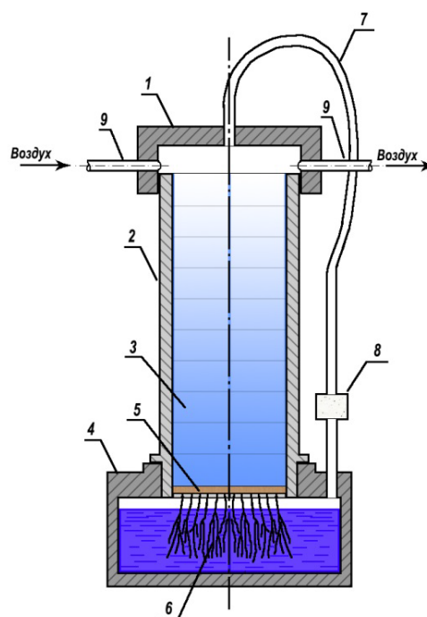
Рис. 37. Схема экспериментального определения влагопроводности стационарным методом:
