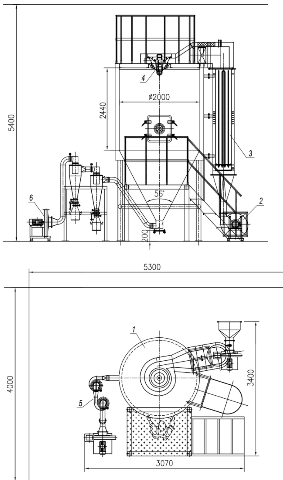
Рис. 113. Распылительная сушилка для сушки раствора ПВП:
