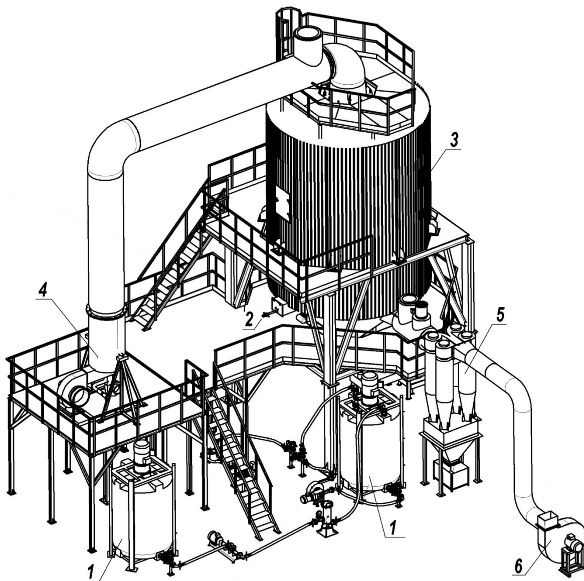
Рис.73. Башенная распылительная сушильная установка:
