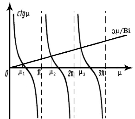
Рис. 31. Корни \mu характеристического уравнения (6.39)
