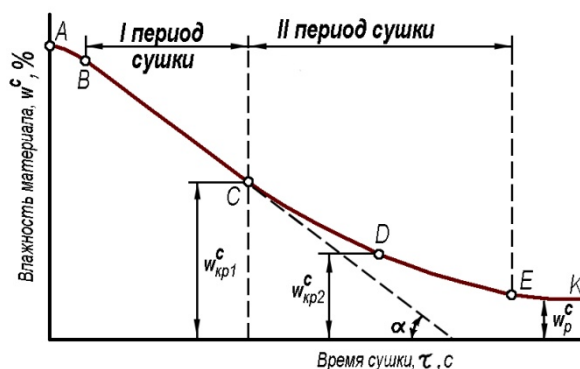
Рис. 25. Кривая сушки материала
