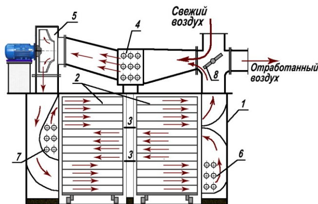
Рис.48. Камерная сушилка: 1 - сушильная камера, 2 - вагонетки, 3 - козырьки, 4, 6, 7 - калориферы, 5 - вентилятор, 8 - шибер
