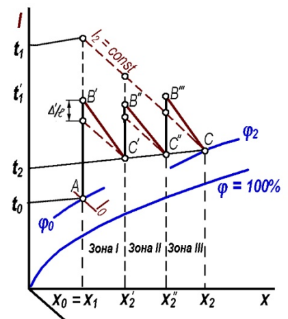
Рис. 18. Изображение процесса реальной сушки с промежуточным подогревом воздуха по зонам.
