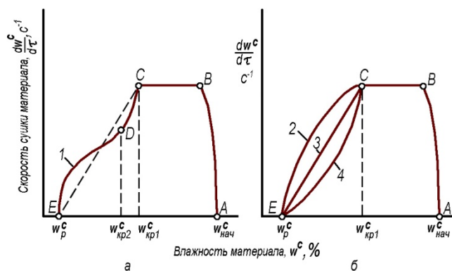
Рис. 27. Вид кривых сушки для различных материалов
