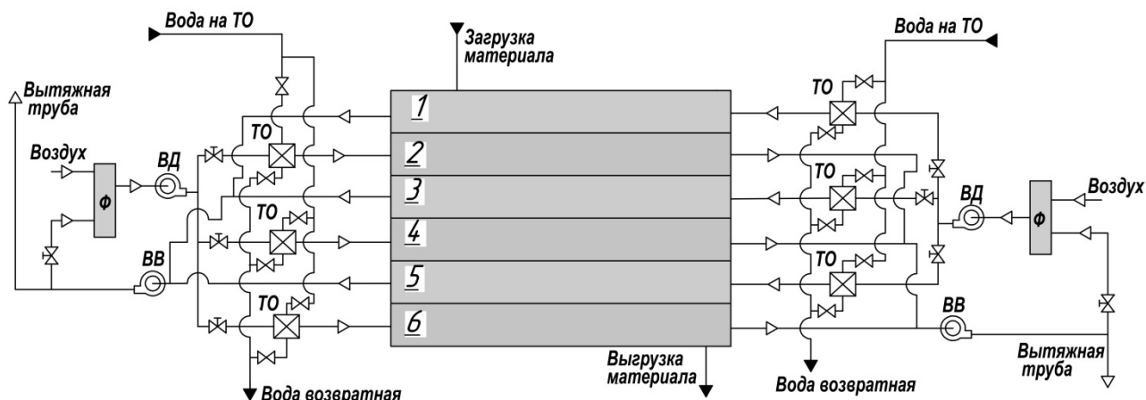
Рис. 115. Схема потоков шестиярусной ленточной сушилки:
