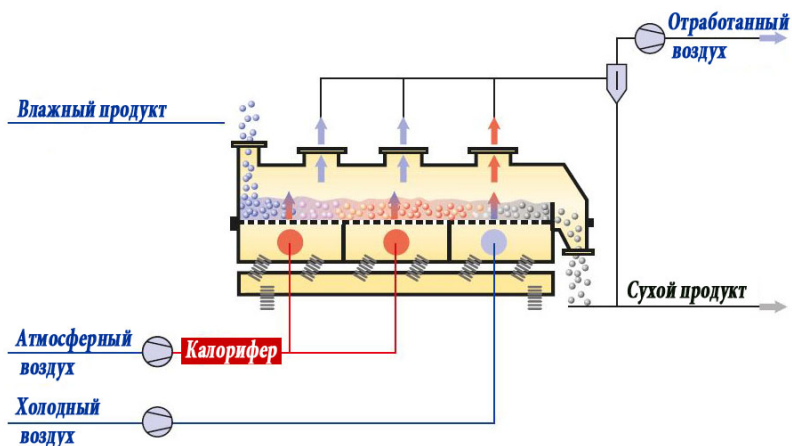
Рис. 71. Вибросушилка с охлаждением продукта на конечной стадии сушки
