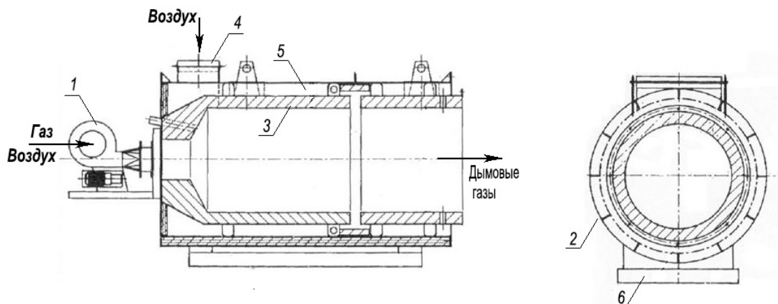
Рис. 105. Схема топки:
