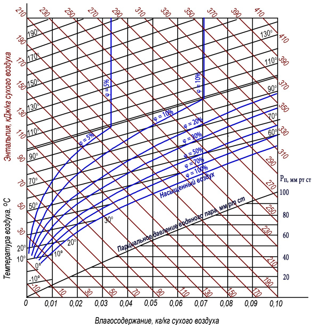
Рис. 6. Диаграмма I - x для влажного воздуха
