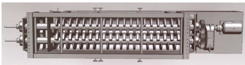
Рис. 83. Сушилка с клиновыми полыми лопастями: 1 - корпус сушилки, 2 - паровая рубашка, 3 – полые лопасти, 4 – полый вал, 5 – инспекционные люки
