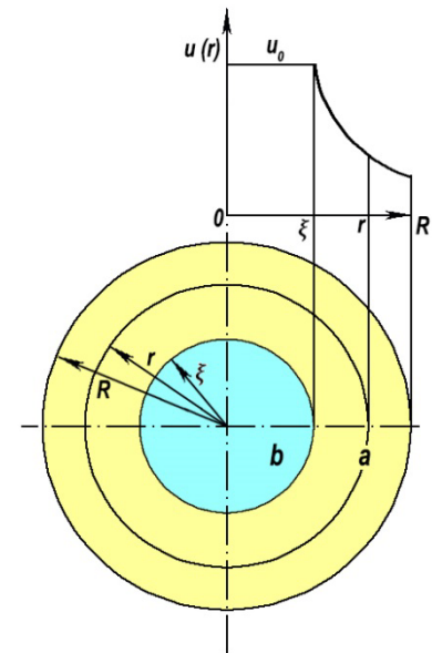
Рис. 35. Схема послойного продвижения фронта испарения при сушке шара: a - сухая зона; b – влажная зона
