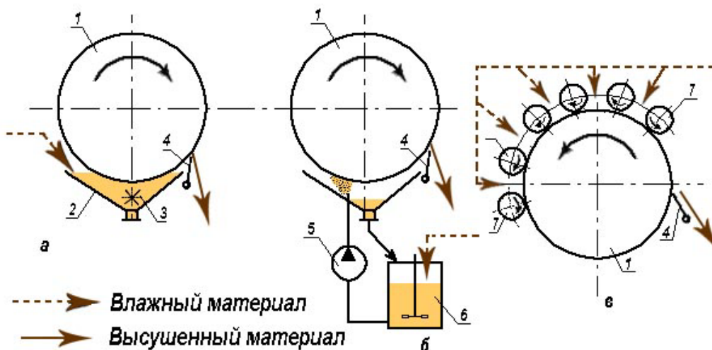
Рис. 88. Способы подачи высушиваемого материала на поверхность вальца: а) из корыта с мешалкой, б) насосом с распылением на валец, в) через смачивающие валики, 1-валец; 2- корыто; 3-мешалка; 4- нож; 5- насос; 6- емкость с мешалкой; 7- смачивающие валики
