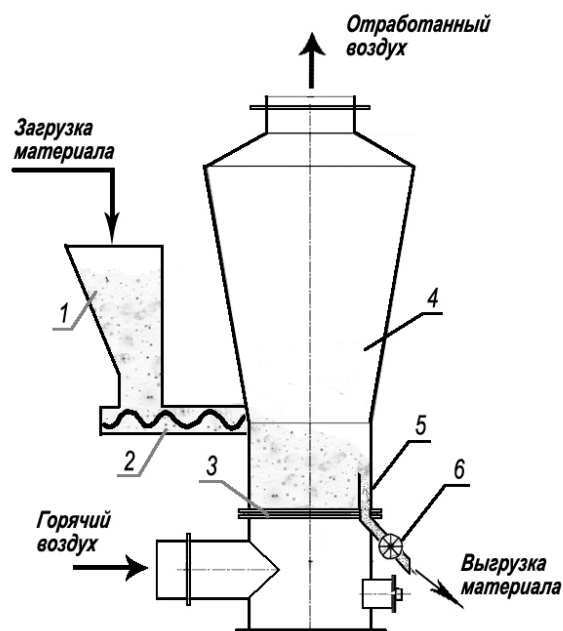
Рис. 64. Сушилка с кипящим слоем материала: 1 - бункер, 2 - питатель, 3 - газораспределительная решетка, 4- камера сушилки, 5 - штуцер для выгрузки высушенного материала, 6 – шлюзовый затвор
