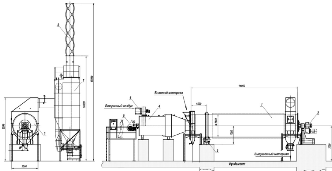
Рис. 102. Промышленная установка для сушки золы ТЭЦ: 1 – сушильный барабан, 2 – привод барабана, 3 – бандаж и опорные ролики, 4 - топка, 5 – горелка, 6 – вентилятор вторичного воздуха, 7 – рукавный фильтр, 8 – дымовая труба (вытяжной вентилятор за фильтром не показан)
